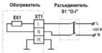
Рис. 2 Схема подключения обогревателя НС-0.8, НС-1.0
