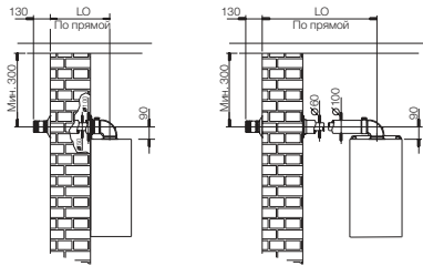
Горизонтальный коаксиальный дымоход
