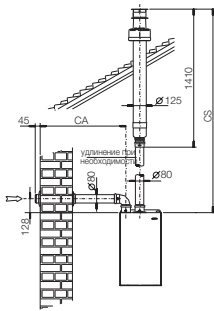
Раздельная система воздухозабора и вертикальным дымоходом.
