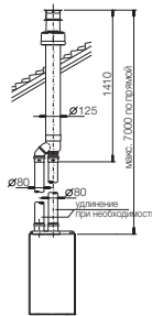
Раздельная система воздухозабора и дымохода с вертикальным коаксиальным дымоходом.
